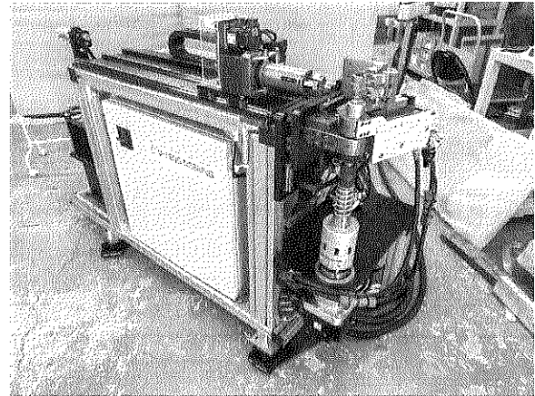
発売中のCNCパイプベンダー「UIB-10型」
